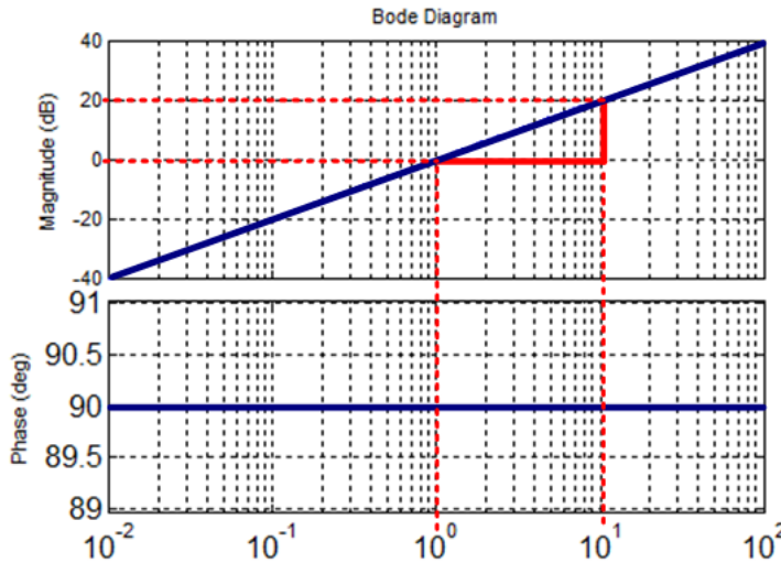
(jw) için Bode çizimi.
